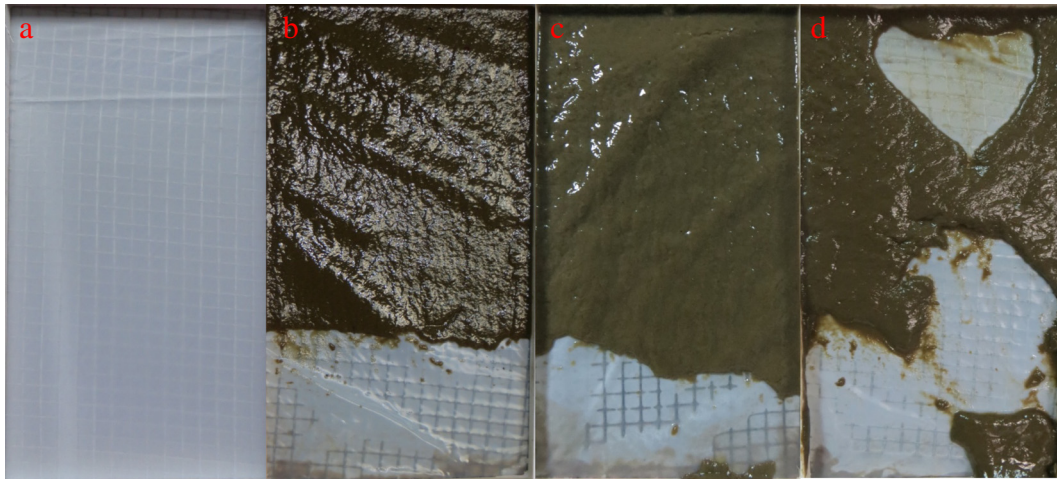
Fig. 5 – Pictures of DM module: (a) new membrane, (b) DM layer of sludge A, (c) DM layer of sludge B, and (d) DM layer of sludge C.
